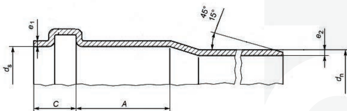
Рисунок 1. Размеры раструбов и трубных концов.
